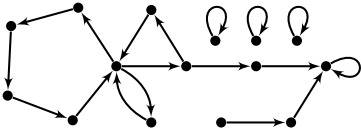
Fig. 12. Graph G_9 .
