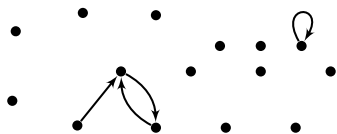
Fig. 19. Graph G_2 .
