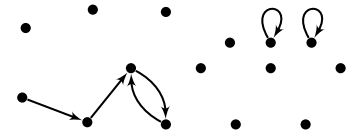
Fig. 18. Graph G_3 .
