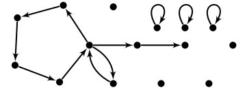
Fig. 15. Graph G_6 .
