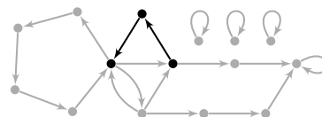
Fig. 10. Path P_3 .
