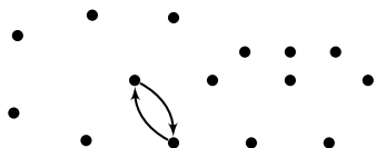
Fig. 20. Graph G_1 .
