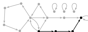
Fig. 8. Path P_2 .
